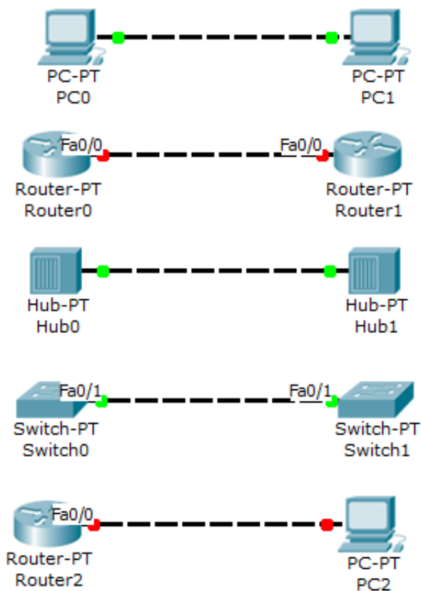
Cable CRUZADO
